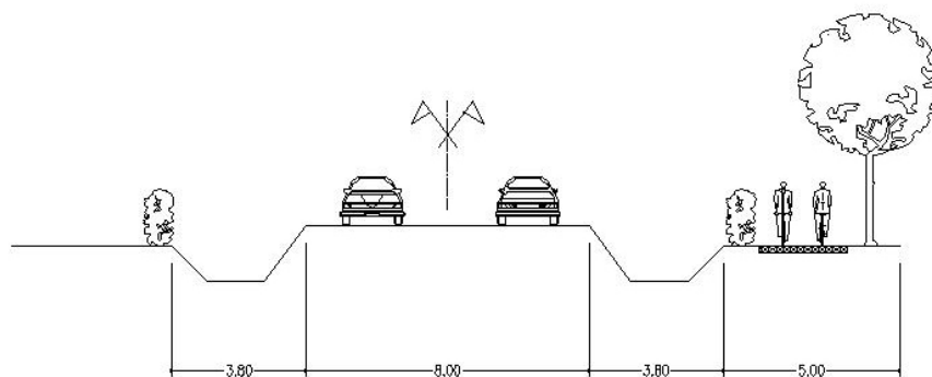
SEZIONE 5 S.P. N. 64, via C. Colombo
