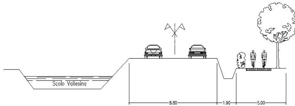
SEZIONE 3 S.P. n. 64, via G. Galilei
