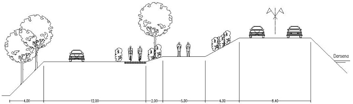
SEZIONE 19 via Po di Venezia
