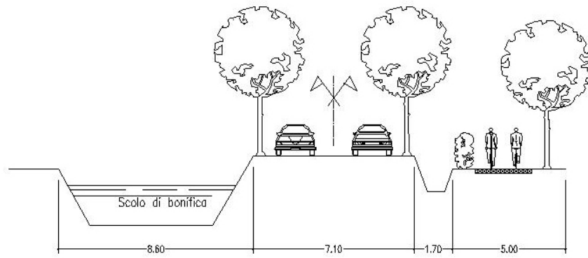
SEZIONE 13 via Ca Pisani
